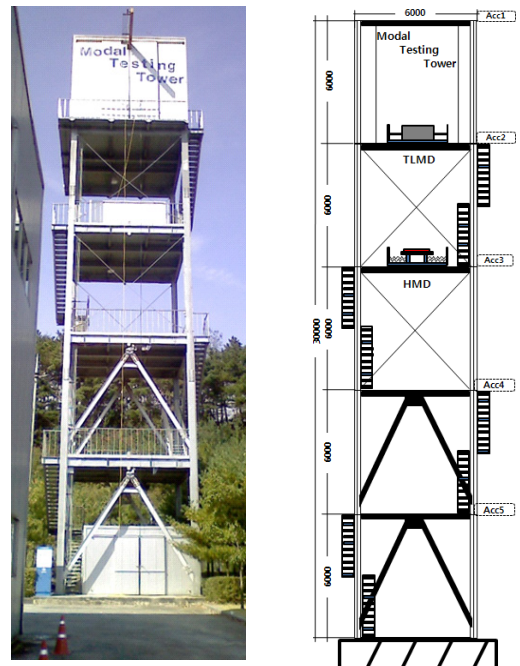
(a) 실험 구조물 사진 (b) 구조물의 정면도
