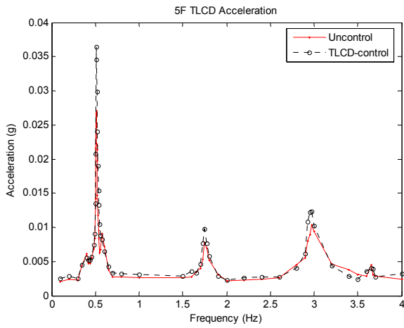
그림 12. TLCD방향 진동수별 5층 가속도 최대 응답 이력
