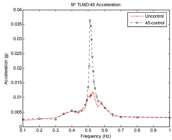
그림 14. TLCD+TMD(45도) 진동수별 5층 가속도 최대 응답 이력
