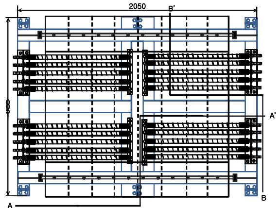
(a) TLMD 투영도
