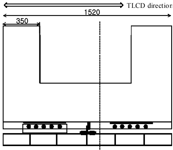
(c) TLMD의 B-B 단면 그림 5. TLMD 상세도
