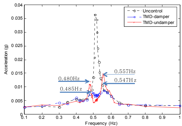
그림 16. TMD_damper와 TMD_undamper 제어성능 평가 비교 (5층)
