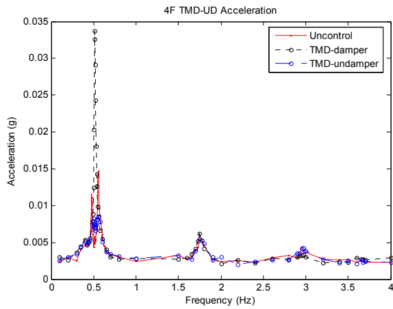
그림 11. TMD방향 진동수별 4층 가속도 최대 응답 이력
