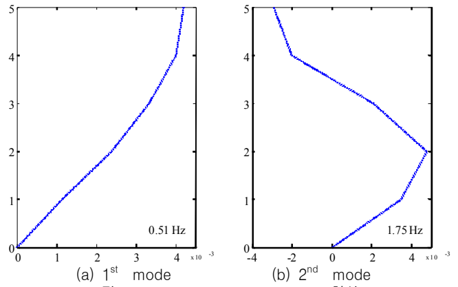
그림 3. Modal Testing Tower 모드 형상
