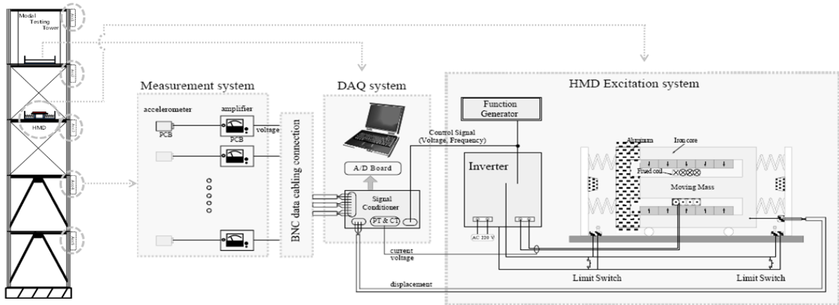
그림 8. 가진시스템 실험 개념도
