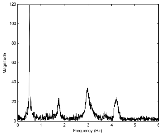
그림 2. Modal Testing Tower 5층 천장 가속도 전달함수
