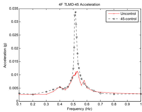
그림 15. TLCD+TMD(45도) 진동수별 4층 가속도 최대 응답 이력
