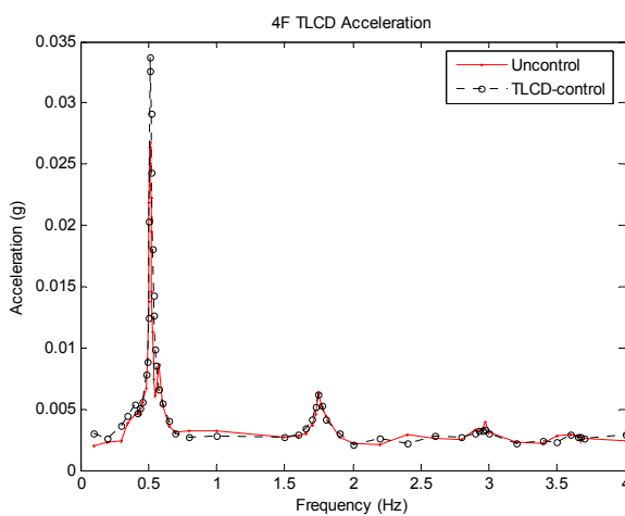
그림 13. TLCD방향 진동수별 4층 가속도 최대 응답 이력
