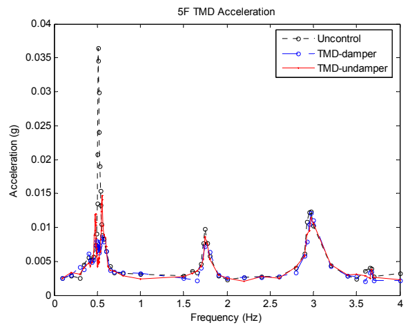
그림 10. TMD방향 진동수별 5층 가속도 최대 응답 이력
