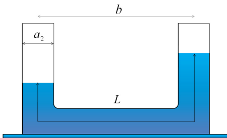
(a) TLCD 정면도
