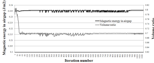
<그림 3> History diagram of Magnetic energy and volume ratio using one steel
