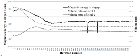
<그림 5> History diagram of Magnetic energy and volume ratio using two steels
