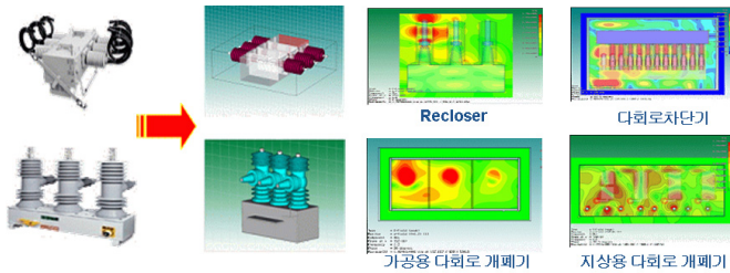
〈그림 1〉 배전기기 Simulation
