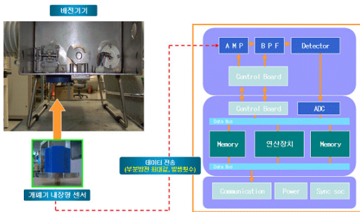
<그림 6> 상태 감시 모듈의 기본 구조
