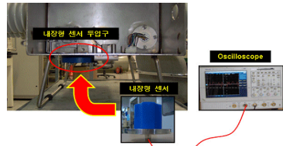
(b) 오실로스코프를 이용한 내장형 센서 성능 테스트 <그림 8> Mock-up 개폐기를 이용한 부분방전 시험
