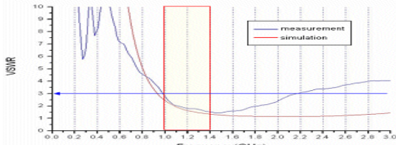
<그림 5> 센서의 VSWR 비교
