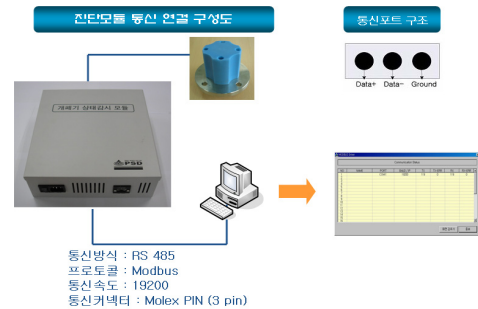
<그림 9> 상태 감시 모듈 데이터 전송 시험
