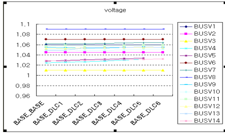
〈그림 1〉 상위 역률 우선 DLC적용 시 모선의 전압
