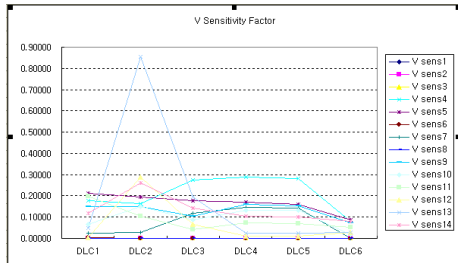
〈그림 3〉 상위 역률 우선 DLC적용 시 전압 민감도
