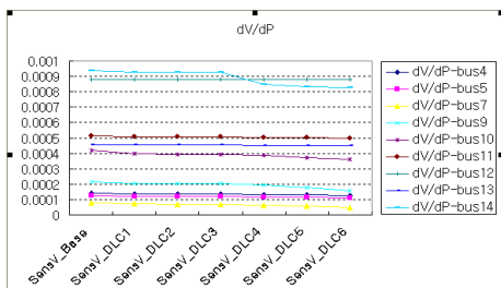
〈그림 5〉 하위 역률 우선 DLC적용 시 조류 민감도
