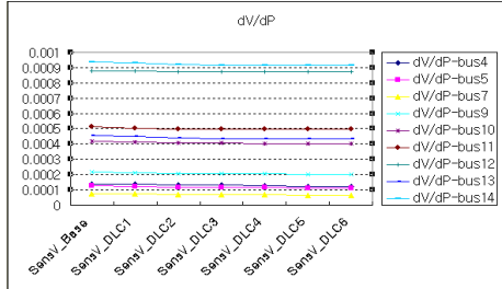
〈그림 2〉 상위 역률 우선 DLC적용 시 조류 민감도
