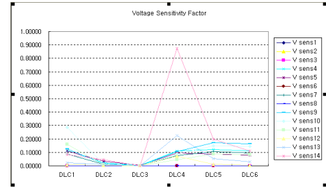
〈그림 6〉 하위 역률 우선 DLC적용 시 전압 민감도
