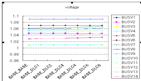
〈그림 4〉 하위 역률 우선 DLC적용 시 모선의 전압
