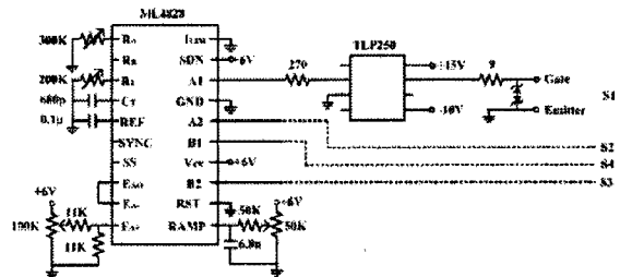
그림 4 제어 회로의 구성도
