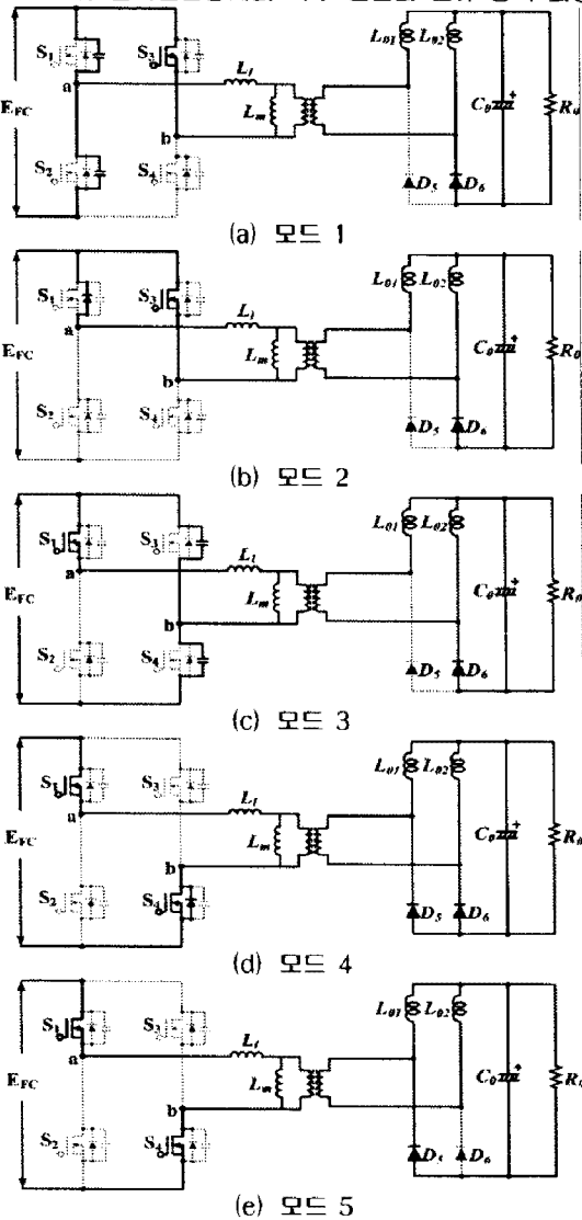
그림 6 제안한 전력변환장치의 1/2주기 동안 동작 모드
