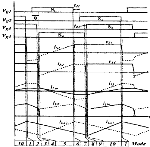
그림 5 제안한 전력변환장치의 각부 전압과 전류 동작 파형
