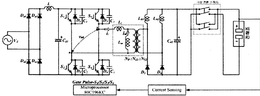
그림 3 제안한 혼합수소가스 발생기용 전력변환장치
