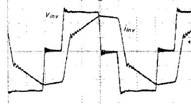
(c) 인버터의 전압과 전류파형 (100 (V/div), 20 (A/div))
