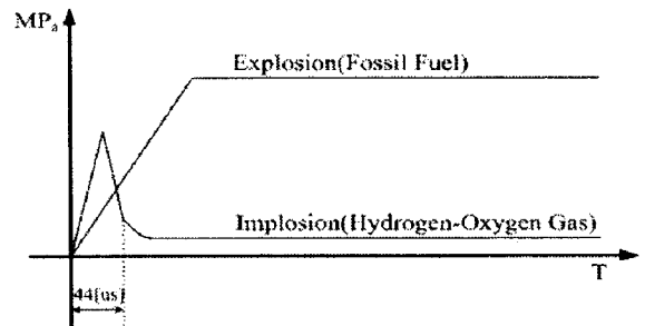
(a) 화석연료와 혼합수소의 폭발시 압력특성
