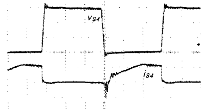
(b) 스위치S4의 전압과 전류파형 (100 (V/div), 20 (A/div))
