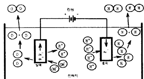
그림 2 물의 전기분해 모식도
