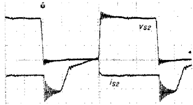
(a) 스위치S2의 전압과 전류파형 (100 (V/div), 20 (A/div))
