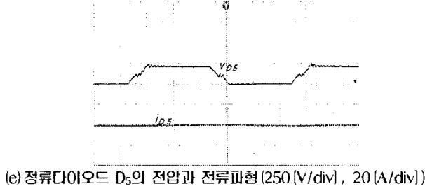
그림 7 무부하시 각부의 전압과 전류파형 (듀티율 최대인 경우)
