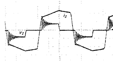
(d) 변압기 2차측의 전압과 전류파형 (250 (V/div), 10 (A/div))
