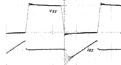
(a) 스위치S2의 전압과 전류파형 (100 (V/div), 10 (A/div))
