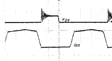
(e) 정류다이오드 D5의 전압과 전류파형 (250 (V/div), 20 (A/div))
