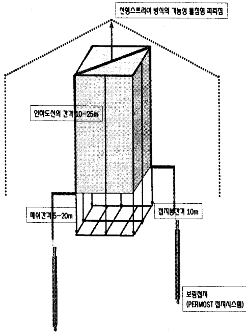
그림 1. 이중보호방식의 예시도
