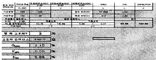
그림 6. 고조파 유출 허용치 산정 프로그램화 3
