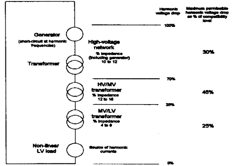
그림 2. 변압기 임피던스에 따른 양립성 레벨의 할당
