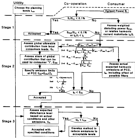
그림 1. IEC 61000-3-6의 고조파 제한 절차
