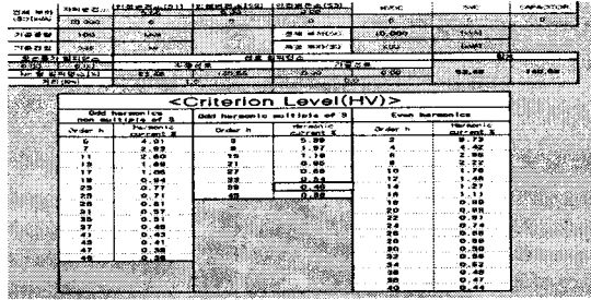
그림 7. 고조파 유출 허용치 산정 프로그램화 4
