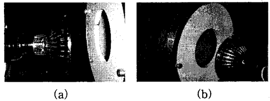
그림 3. 광속구 외부의 측정시료 고정 모습
