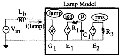
그림 8. 동적 특성을 포함한 형광등의 램프 모델 [2]
