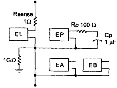
그림 3. 형광등의 PSpice 회로 모델 [1]
