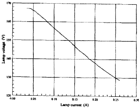
그림 2. T8 형광램프의 전압-전류 특성
