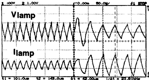
그림 7. 램프 전력이 변할때의 전압, 전류의 파형 변화
