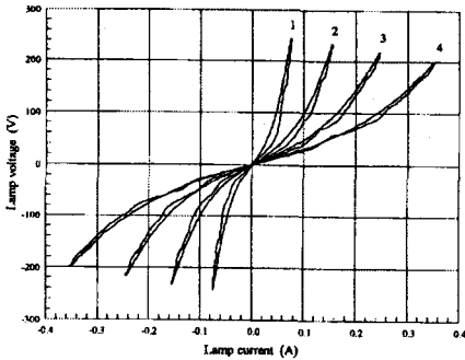
그림 5. 형광등의 여러 램프전력에 대한 동적특성 변화 (램프 전력은 P_4 > P_3 > P_2 > P_1 )
