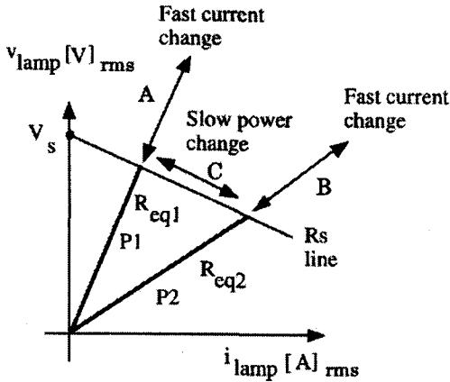
그림 5. 형광등의 동적특성과 정적특성의 관계 ( P_2 > P_1 )
