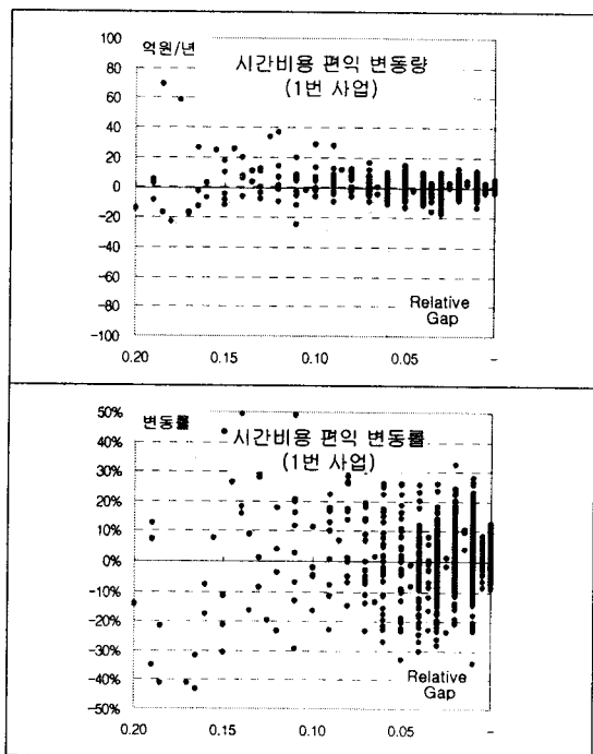
[그림 4] 종료기준(RG)에 따른 통행시간편익의 변동량 및 변동률(1번 사업, RG=0.01~0.20)
