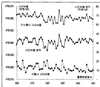
[그림 1] 통행배정횟수에 따른 통행시간비용의 변화(1번 사업)
