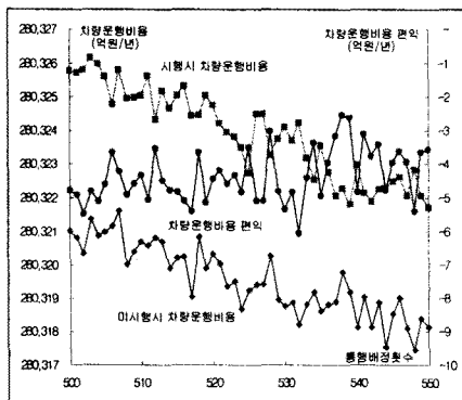
[그림 2] 통행배정횟수에 따른 차량운행비용의 변화(1번 사업)
