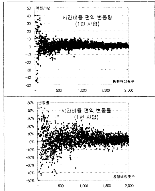
[그림 3] 통행배정횟수에 따른 통행시간편익의 변동량 및 변동률(1번 사업, 1회~2000회)
