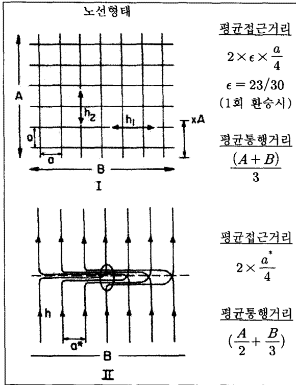
<그림 2> 격자형 가로망에서의 두 가지 노선형태와 각 노선형태에 따른 전체 이용자의 평균 접근거리 및 통행거리 (Newell, 1979)
