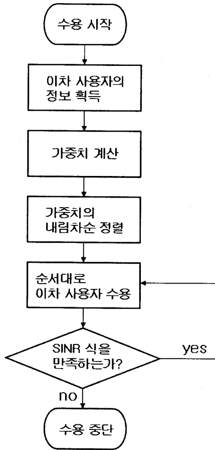
[그림 2] 이차 사용자 수용 알고리즘
