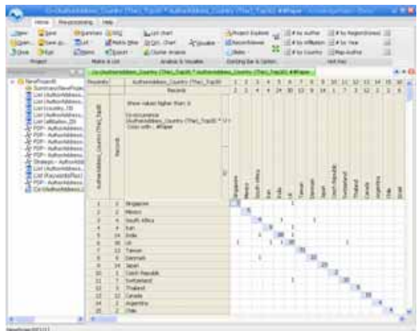
▶▶ 그림 7. Home 전체화면
