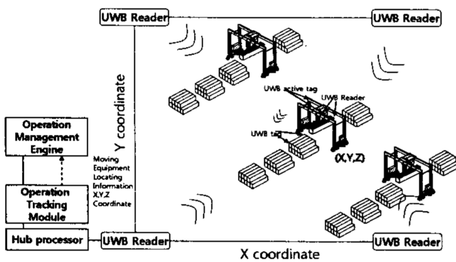
그림 2 UWB를 이용한 야드 크레인 제안모델
