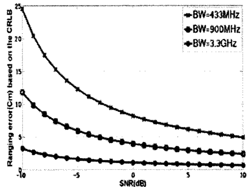
그림 4 Ranging Error
