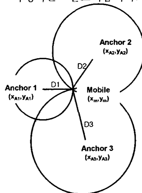
그림 1 ToA 알고리즘
