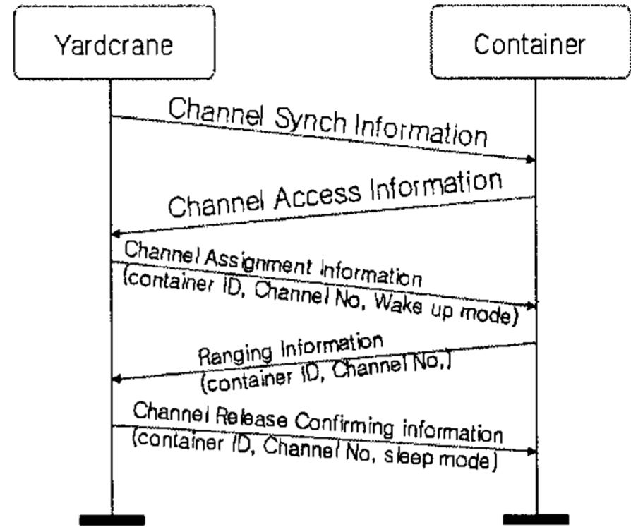
그림 3. 컨테이너와 야드 크레인의 위치추적 흐름도
