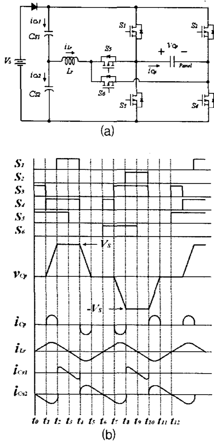
그림 1. 제안된 서스테인 드라이버, (a)회로구성, (b)주요 동작파형
