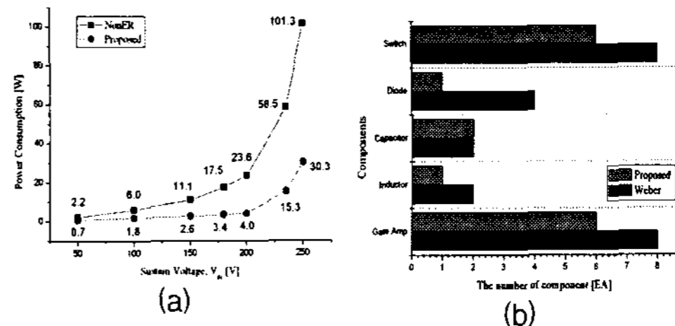
그림 5. 소비전력 및 소자 수 비교, (a)소비전력, (b)소자 수
