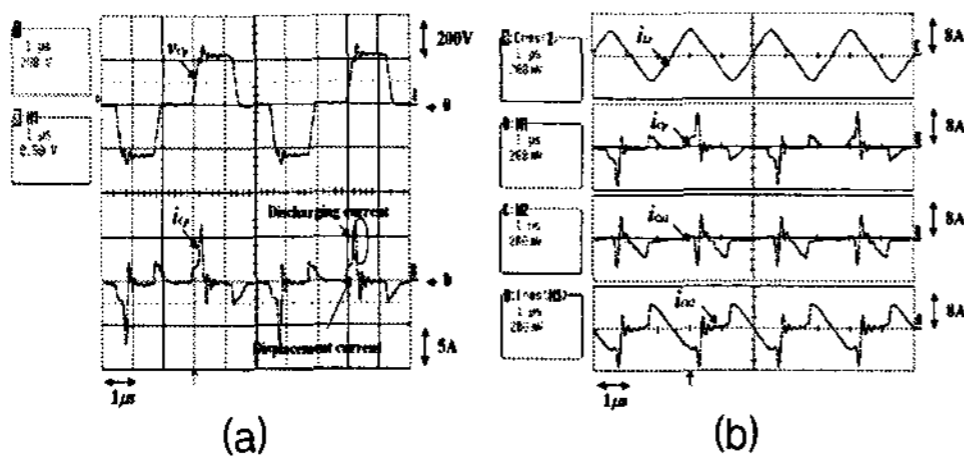
그림 4. 방전 후, (a)패널전압/전류, (b)인덕터, 패널, 콘덴서 전류
