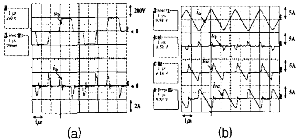
그림 3. 방전 전, (a)패널전압/전류, (b)인덕터, 패널, 콘덴서 전류
