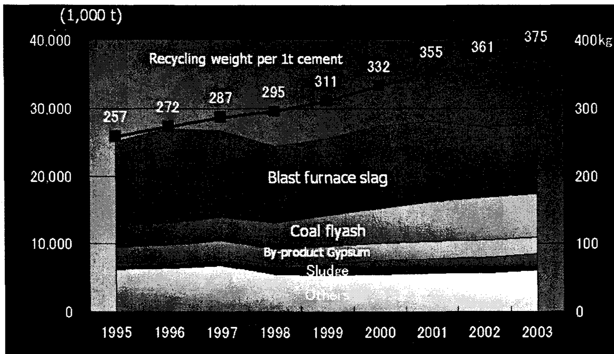
<그림 2> 시멘트 제조 시 폐기물이 차지하는 비율
