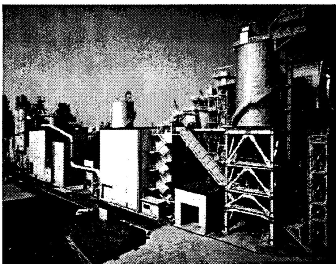
<일본 치바현 Eco-cement plant 전경>
