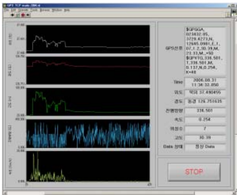
그림 5. GPS 수신프로그램 주화면
