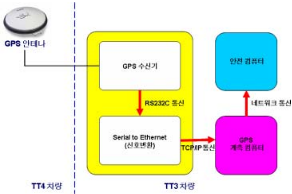
그림 1. GPS 계측시스템 구성도
