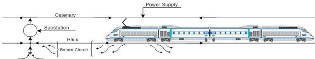
그림 1. 전차선 전류 순환도
