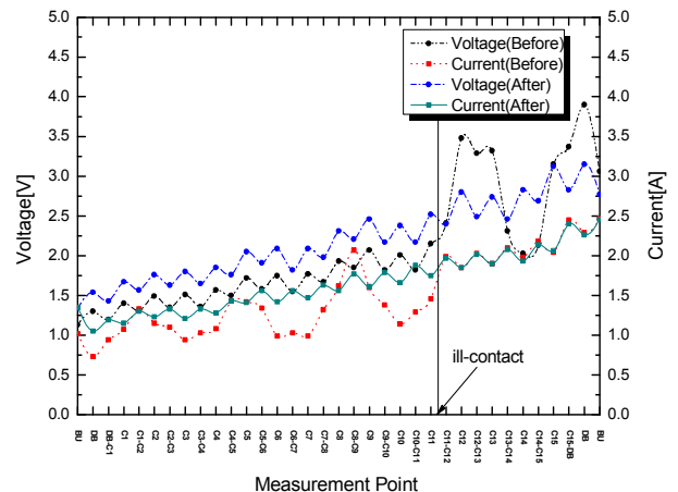
그림 8. TC2053 레일전압 및 단락전류 특성
