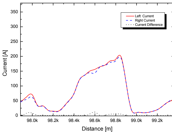
그림 11. 귀선전류(TC2053-조치 후)
