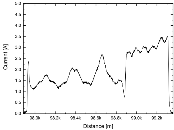
그림 10. 차상신호레벨(TC2053-조치 전)
