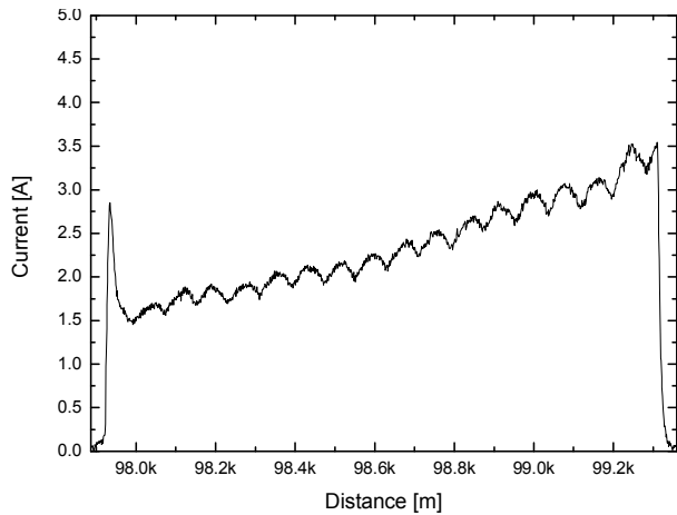
그림 12. 차상신호레벨(TC2053-조치 후)
