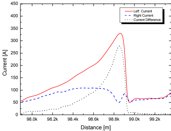
그림 9. 귀선전류(TC2053-조치 전)
