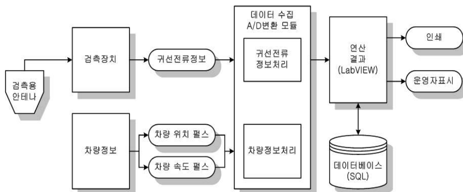
그림 4. 귀선전류 검측시스템 구성도
