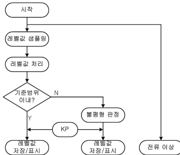
그림 5. 귀선전류 불평형 정보처리 알고리즘
