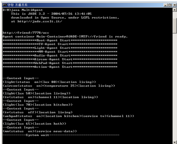
그림 5. 상황정보에 따라 추론된 메시지
