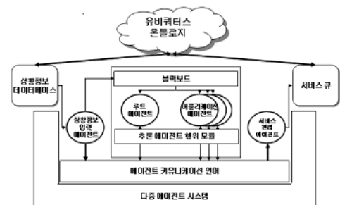
그림 4. 다중 에이전트 시스템의 구조
