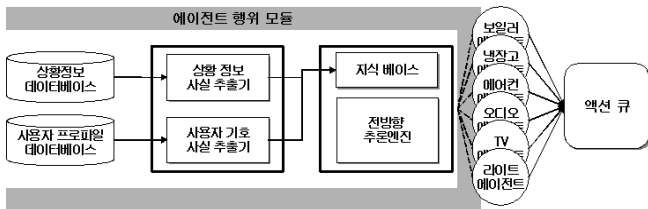
그림 1. 추론엔진이 적용된 에이전트 행위 모듈 구조
