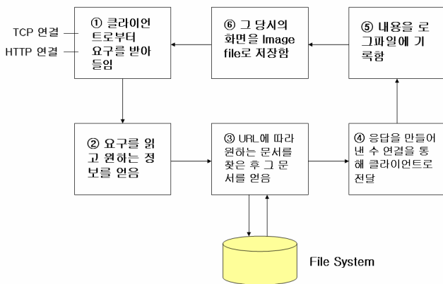
<그림 1> Image Logging Web Server의 알고리즘
