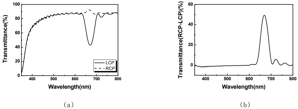
그림 1. 나선형 구조로 증착된 TiO 2 박막의 (a) 원편광에 따른 투과 스펙트럼, (b) 원편광에 따른 투과 스펙트럼 차이
