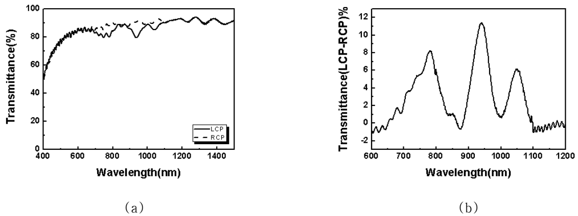
그림 2. 나선형 구조로 3-밴드를 가진 TiO 2 박막의 (a) 원편광에 따른 투과 스펙트럼, (b) 원편광에 따른 투과 스펙트럼 차이
