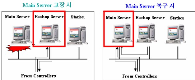
그림 4. 서버 이중화 기능
