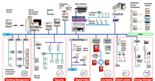
그림 1. EBI 통합시스템 구성도
