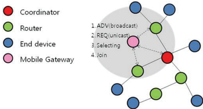
<그림 3> Gateway 가 ZigBee 노드와 join 하는 과정
