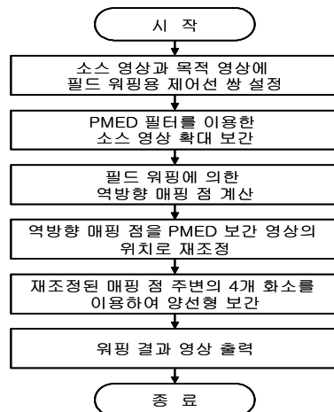
그림 1. 제안된 방법의 순서도
