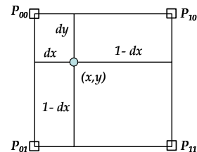
그림 3. 양선형 보간의 화소 위치
