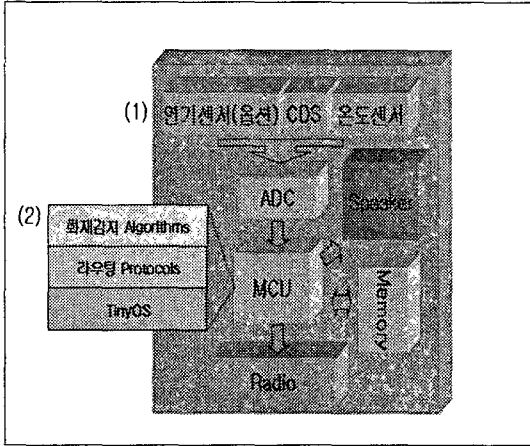
그림 4. 무선 화재감지/경고 모듈
