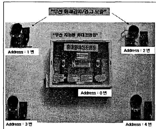
그림 8. 실험을 위해 제작된 무선 지능형 화재 감지/경고 시스템
