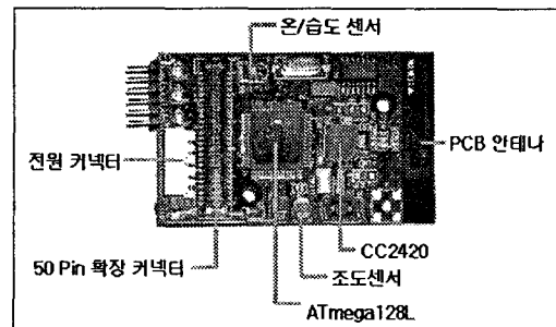
그림 6. Zigbex 메인보드
