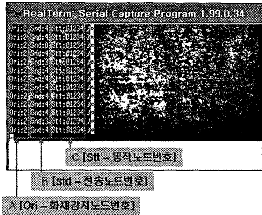
그림 9. flooding에 의한 동작 테스트 화면
