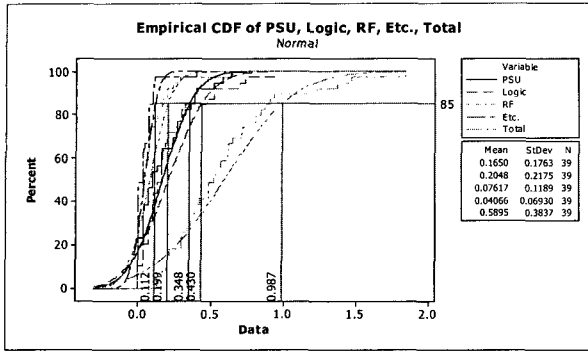
<그림 4> 경험적 누적분포함수(CDF)에 의한 고장률
