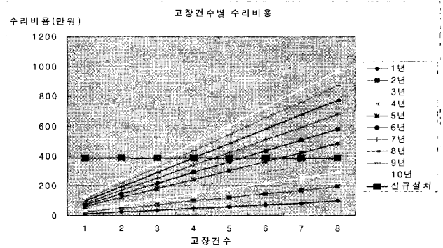
<그림 5> 고장건수에 의한 비용곡선
