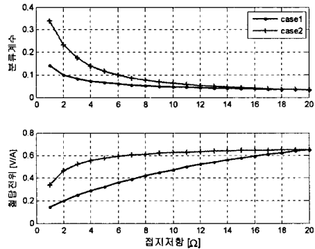
그림 2. 접지 분류계수 및 단위 지락전류에 대한 탐각전위
