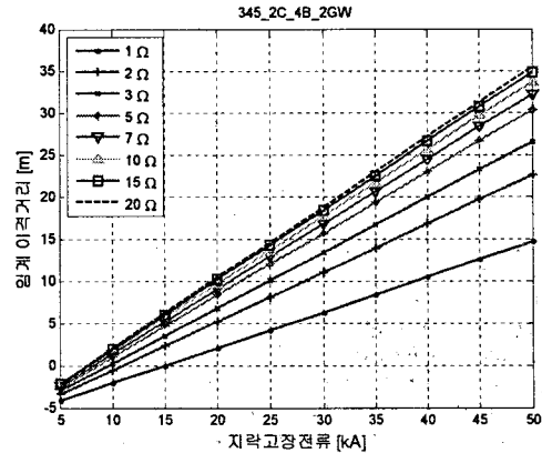
그림 6. 고장전류 크기 및 탐각저항별 이격거리 계산사례
