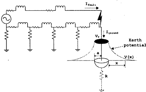
그림 5. 대지전위 계산을 위한 회로-반구전극 합성모델
