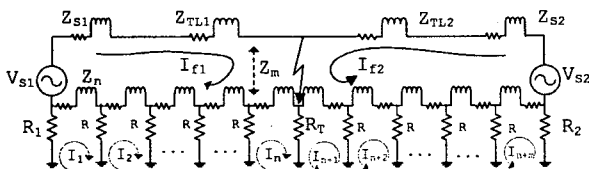
그림 1. 송전선 지락시 접지전류 계산모델
