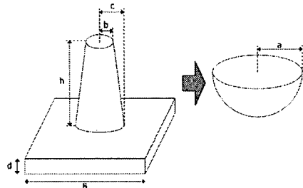
그림 3. 탐각 기의 등가 반구 모델
