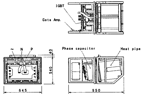
〈그림 2〉 컨버터 외형
