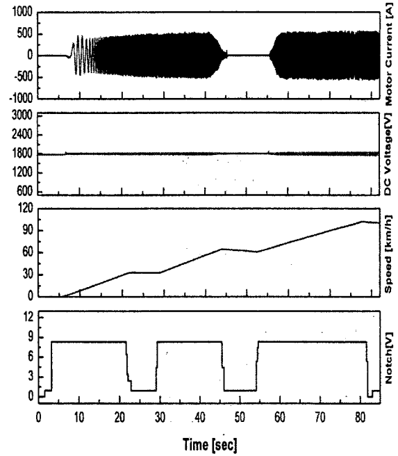
〈그림 6〉 재역행시험
