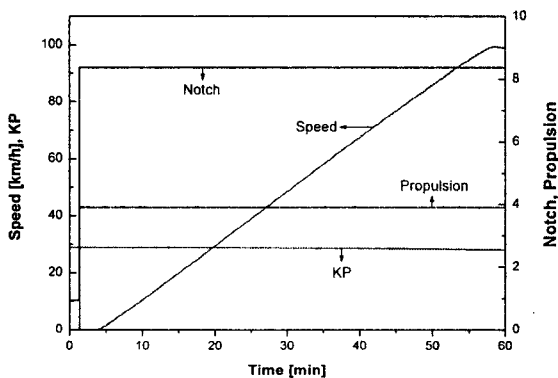
〈그림 5〉 가속도시험
