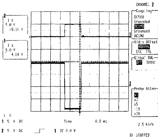
그림 8. 일반적인 호흡할 때의 신호출력 파형
