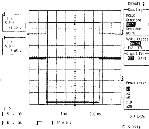
그림 9. 지속적인 압력에 대한 신호출력 파형
