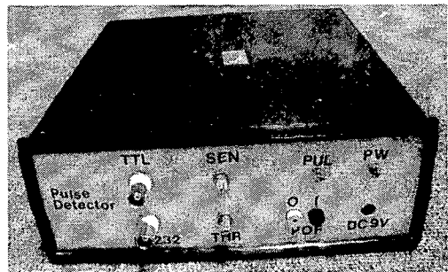
그림 5. 센서 수신부의 외관도
