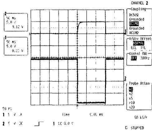
그림 7. 손을 움직였을 때의 신호출력 파형
