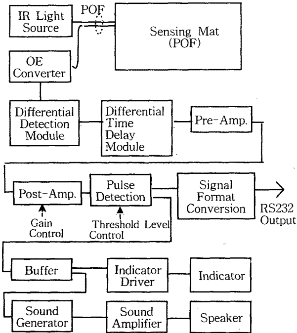
그림 3. 의료용 센서 매트 센서부 블록도
