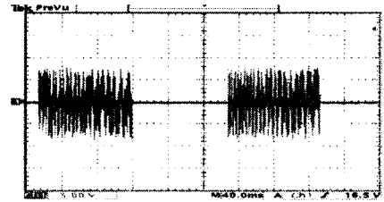
Fig 6. (pulse 2차, gap 10ms, with: 100ms)
