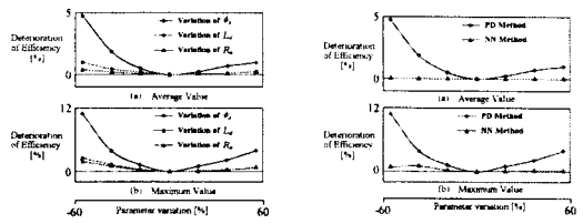
그림 9 파라미터 변동에 대한 효율 감소율 ( i_{dopt} = PD )
