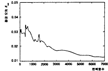
그림 4 신경회로망의 평균 절대오차
