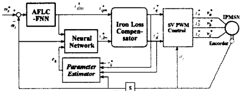
그림 2 효율 최적화 제어를 위한 드라이브 시스템
