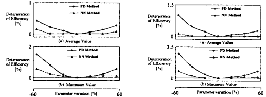
그림 10 파라미터 변동에 대한 효율 감소율 비교 ( \phi_s = \pm 0.6\phi_s )
