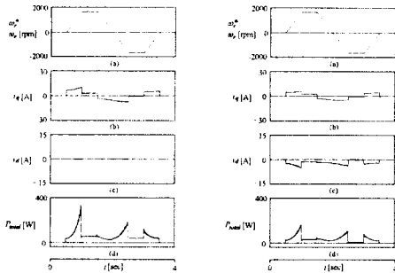
그림 5 4상한 운전의 대한 응답 특성 ( i_{d0} 제어)
