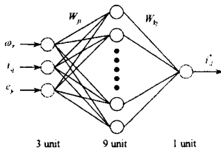
그림 3 최적 d 축 전류의 동정을 위한 신경회로망
