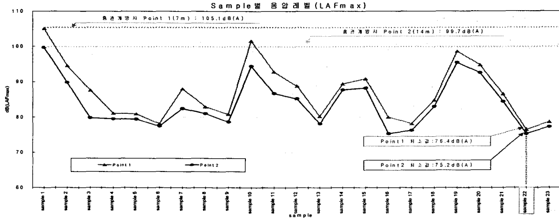
그림 9. 방음재질별 LAFmax에 의한 음압레벨
