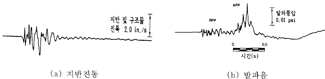
그림 1. 동일발파로 인한 지반진동과 발파음의 시간이력 특성
