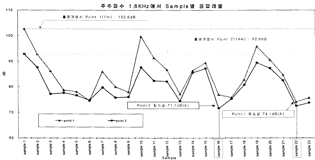
그림 12. 주주파수 대역(1.6KHz)에서의 방음재질별 음압레벨
