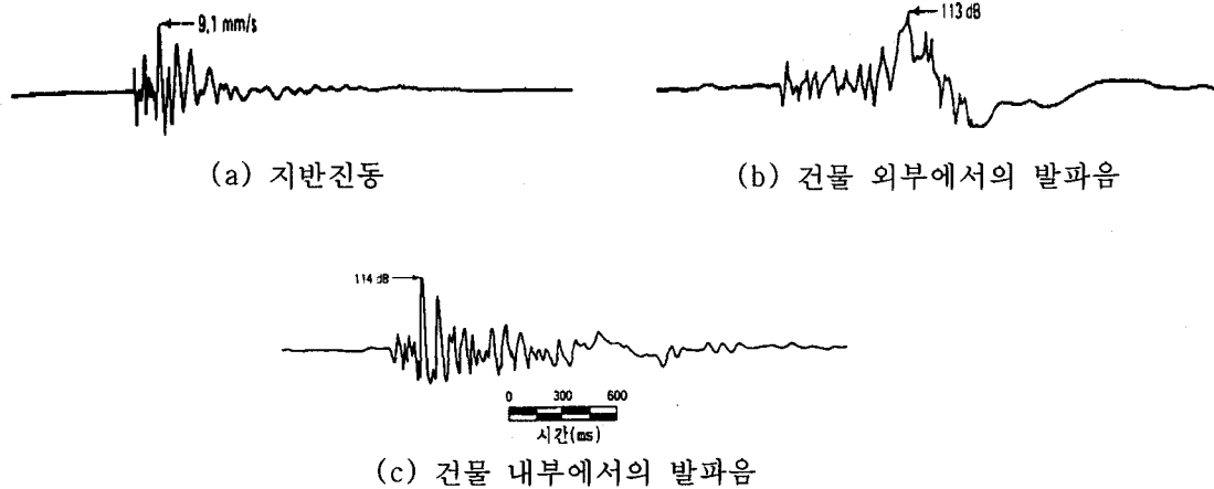
그림 2. 건물 내·외부에서의 발파소음
