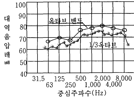
그림 4. 옥타브대역 음압레벨
