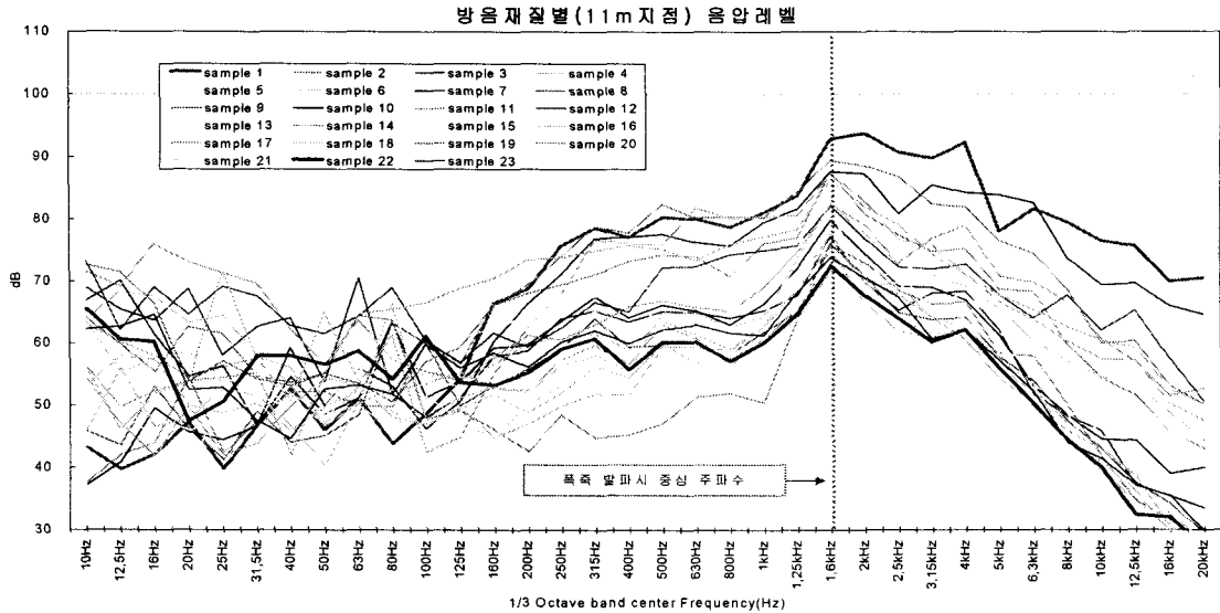
그림 11. 폭죽소음에 의한 방음재질의 주파수 대역별 음압(11.0m)
