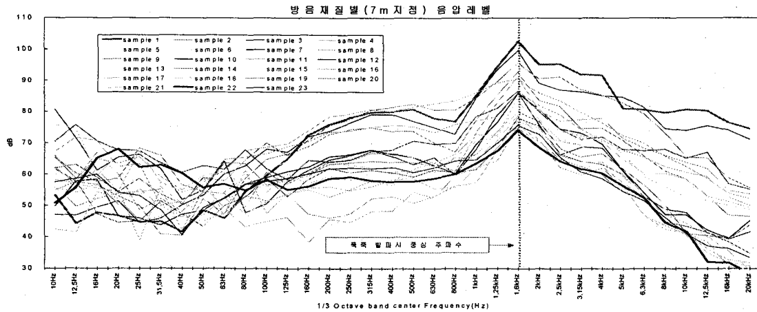
그림 10. 폭죽소음에 의한 방음재질의 주파수 대역별 음압(7.0m)
