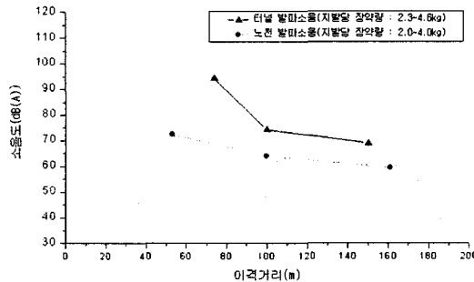
그림 3. 동일지역의 터널 및 노천발파 소음 계측사례
