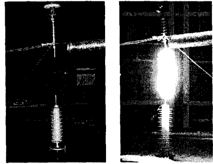
그림 2. 50% 섬락전압시험
