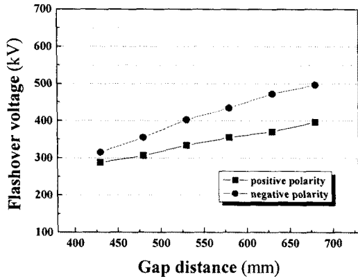
그림 1. 개폐서지 섬락전압 변화
