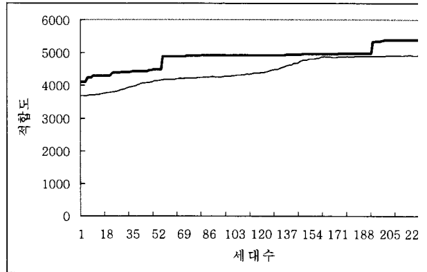
그림 6. 적합도 변화
