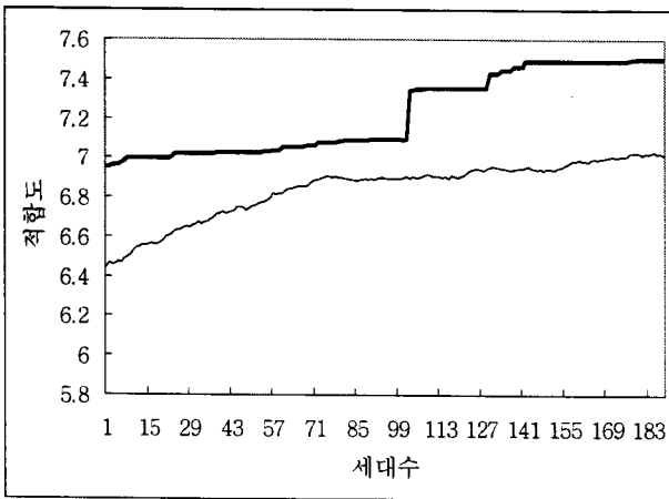
그림 5. 적합도의 변화
