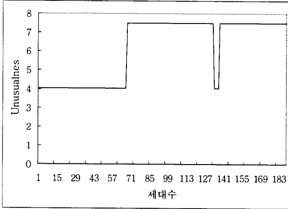
그림 7. Unusualness의 변화
