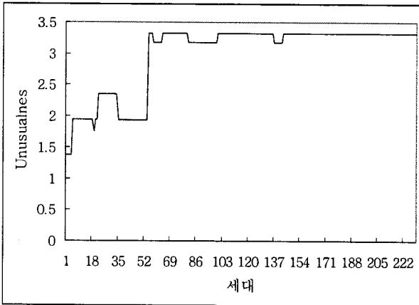
그림 8. Unusualness의 변화
