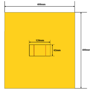
(a) 정면도
