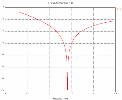
(a) S 11 Parameter (0.3~2.5[GHz])
