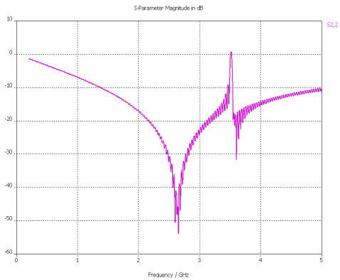
(c) S 22 Parameter (0.2~5[GHz])
