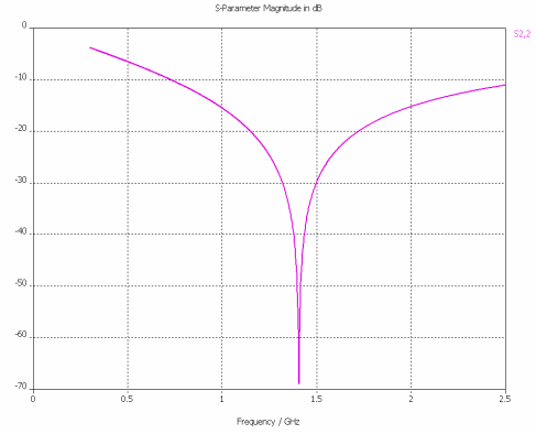
(b) S 22 Parameter (0.3~2.5[GHz])
