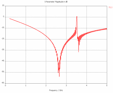
(b) S 11 Parameter (0.2~5[GHz])
