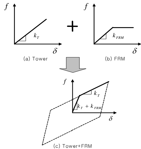
그림 11. 마찰형 보강기구의 거동 형상
