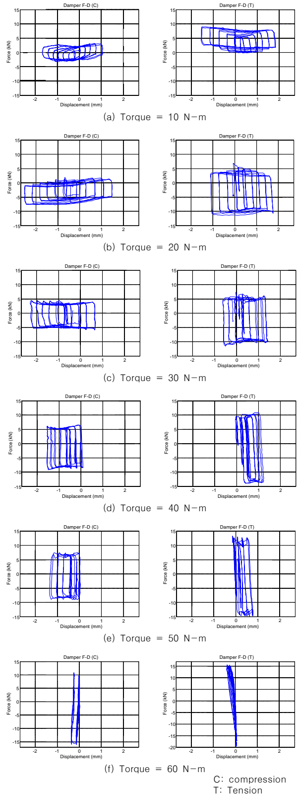
그림 15. 마찰형 보강기구의 슬롯볼트형 접합부의 축력-상대변위 관계
