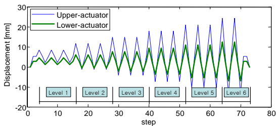
그림 9. 반복하중 강제변위
