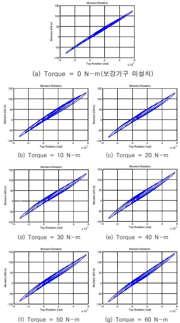
그림 14. 모멘트-회전각 곡선
