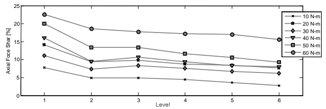
(a) 압축력 분담률
