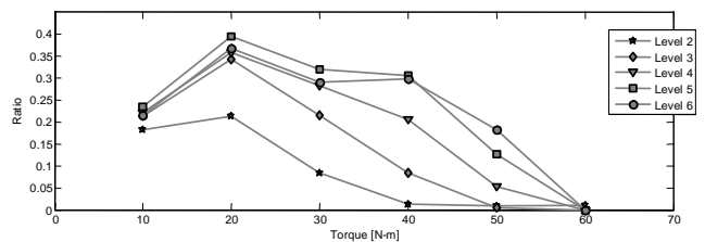
그림 18. 전체 에너지 소산량에서 슬롯볼트형 마찰감쇠기가 차지하는 비중
