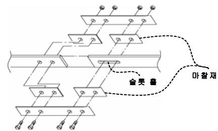
(a) 마찰형 감쇠기 상세
