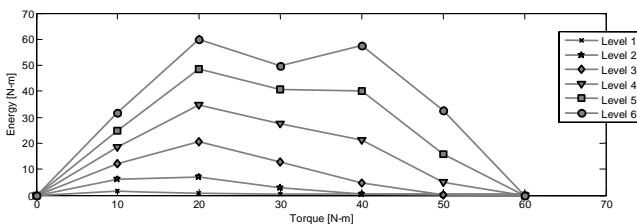
그림 16. 슬롯볼트형 마찰감쇠기의 에너지 소산량
