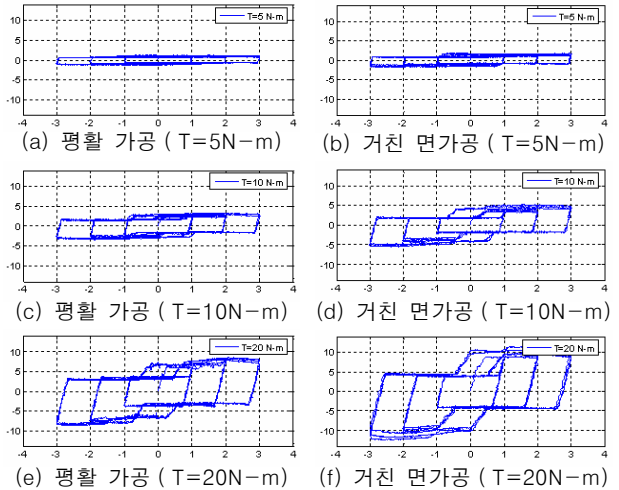
그림 4. 아연도금 강판과 황동판을 사용한 마찰형 감쇠기의 토크 별 하중-변위 곡선
