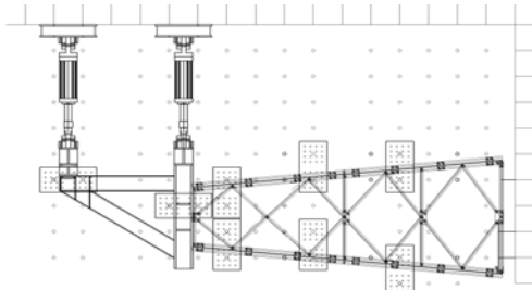
그림 7. 실험체 및 가력기 구성도
