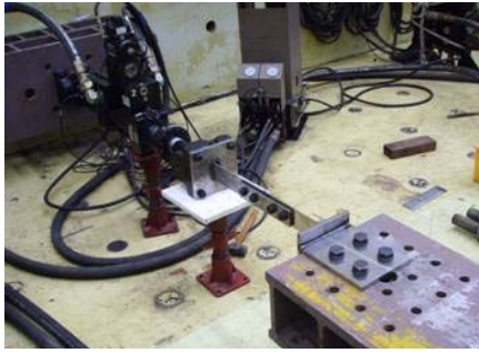
(c) 특성시험 전경 그림 2. 마찰형 감쇠기 특성시험
