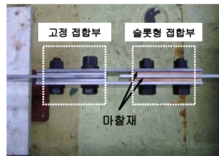
(b) 마찰형 감쇠기 형상 그림 2. 마찰형 감쇠기 특성실험
