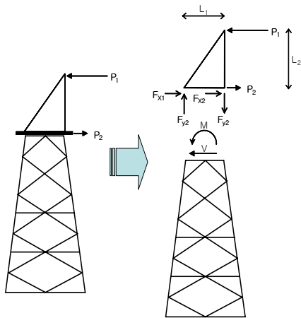
그림 8. 지그 반력에 의한 하중 전달
