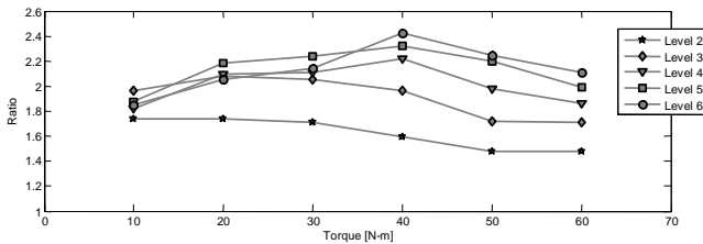
그림 19. 마찰형 보강기구 설치 이전과 비교한 전체 에너지 소산량 증가율
