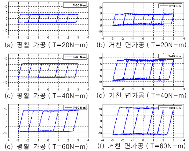
그림 3. 일반 강판과 황동판을 사용한 마찰형 감쇠기의 토크 별 하중-변위 곡선
