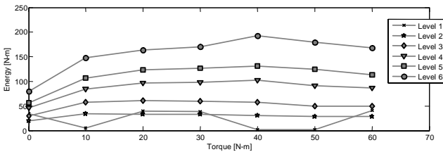
그림 17. 실험체 전체의 에너지 소산량
