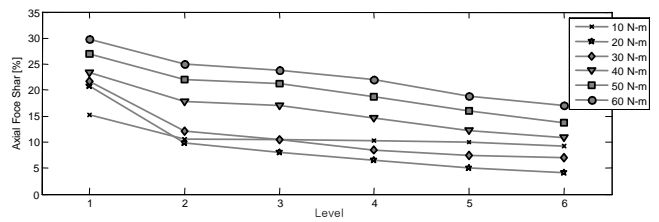
(b) 인장력 분담률
