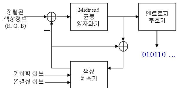
그림 1. 제안한 색상 부호기의 블록도
