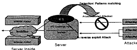
[그림 5] IPS의 기본 구조
