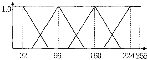
그림 2. R,G,B 각각의 소속함수
