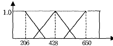
그림 3. X좌표의 소속 함수
