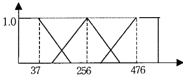
그림 4. Y좌표의 소속 함수
