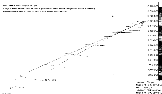
Fig. 7 고유진동 해석 (mdoe-2, 6,176 Hz)
