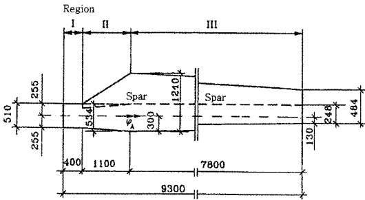
Fig. 2 100kW급 풍력발전기 블레이드 형상
