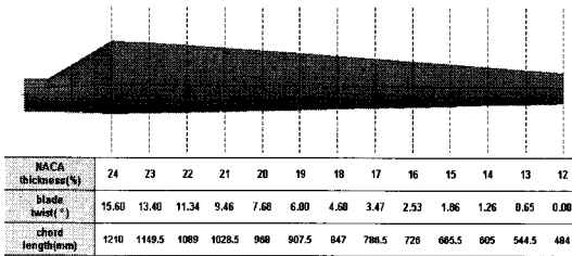
Fig. 3 복합재 블레이드의 단면 형상 정보
