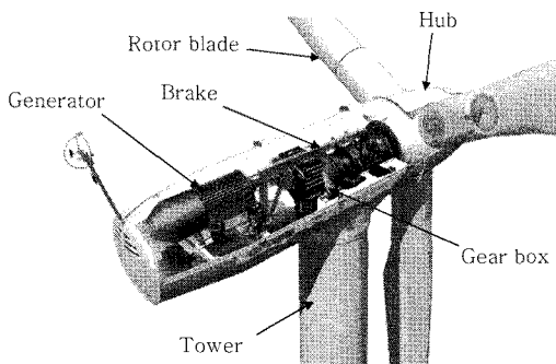
Fig. 1 풍력발전기 시스템
