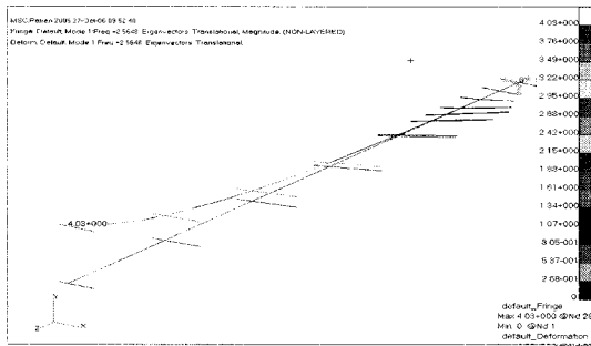
Fig. 6 고유진동 해석 (mode-1, 2,565 Hz)
