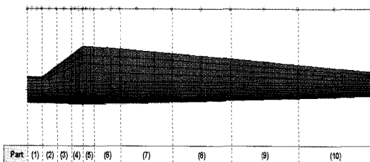
Fig. 4 등가 보 모델의 구성
