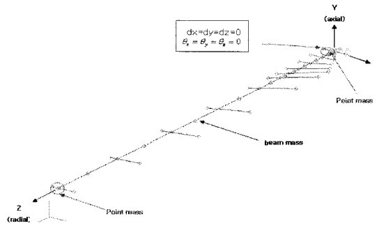
Fig. 5 등가 구조 모델
