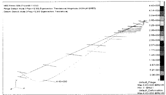
Fig. 8 고유진동 해석 (mode-3, 12,353 Hz)
