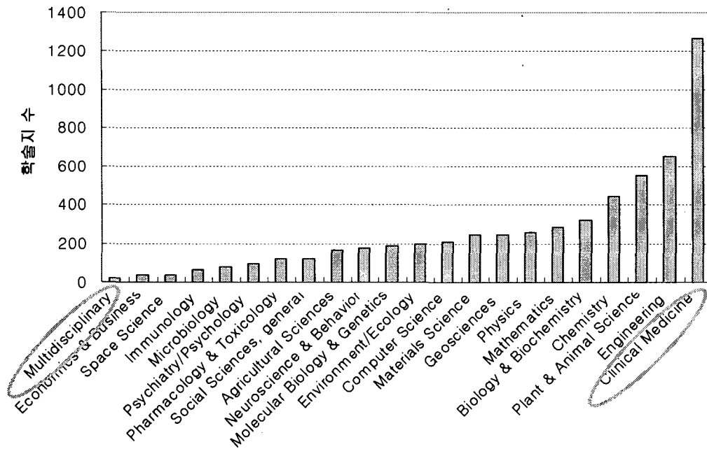
<그림 2> ESI 분류별 학술지 수
