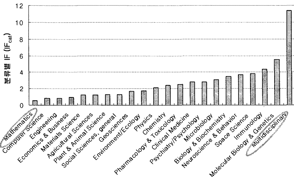
<그림 4> ESI 분류별 IF(IF cat )
