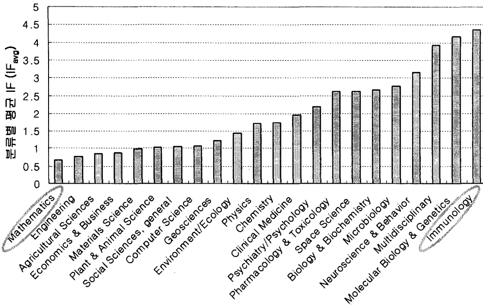
<그림 3> ESI 분류별 평균 IF(IF avg )
