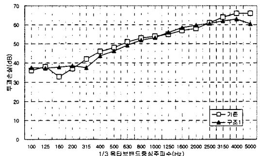
그림 3. 주파수 특성
