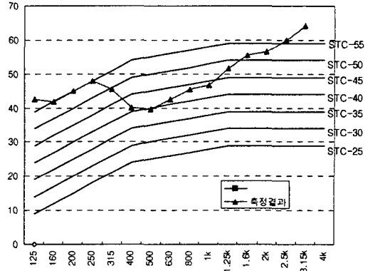
그림 5. STC 곡선에 의한 측정 결과
