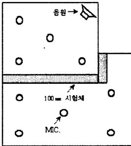
그림 2. 시험체 설치(현장)
