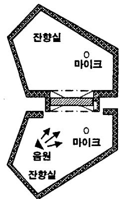
그림 1. 잔향실 시험
