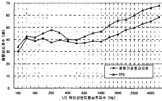
그림 4 주파수 특성
