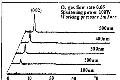
그림 1. 두께 변화에 따른 AZO 박막의 XRD 패턴
