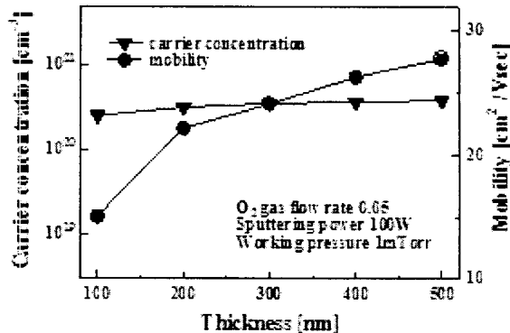
그림 4. 두께 변화에 따른 AZO 박막의 캐리어 농도 및 이동도
