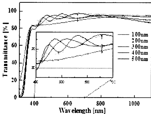
<그림 5> 두께 변화에 따른 AZO 박막의 투과율
