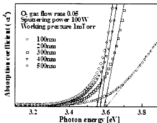
<그림 6> AZO 박막의 흡수율 대 입사에너지
