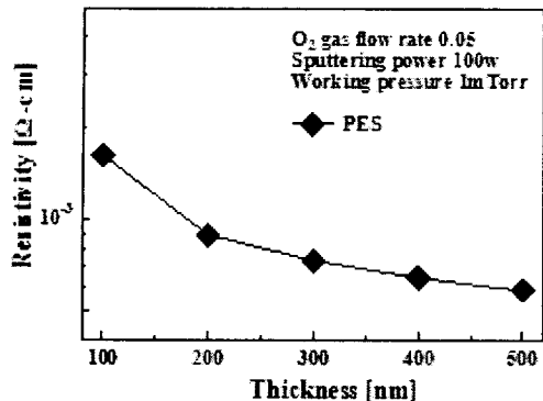
그림 3. 두께 변화에 따른 AZO 박막의 비저항
