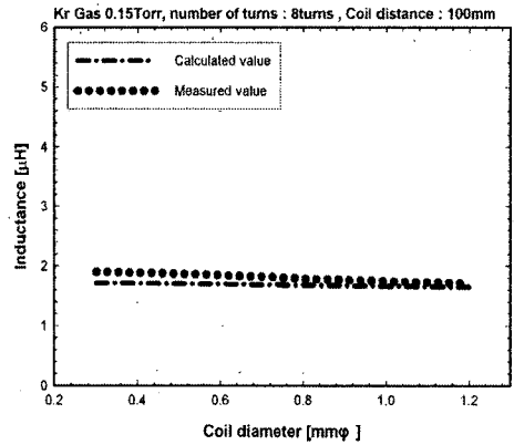
그림 4. 코일의 직경 변화에 따른 인덕턴스 특성.
