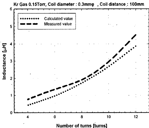
그림 7. 코일의 권선수 변화에 따른 인덕턴스 특성. Fig. 7. Inductance Dependence on Coil turns.
