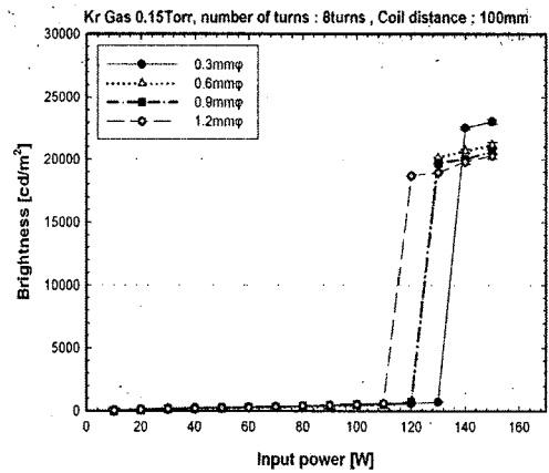
그림 5. 코일의 직경과 RF 전력변화에 따른 휘도 특성.
