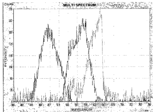
그림 12. 평판형 광원의 스펙트럼 Fig. 12. Spectrum for Lighting-Sources.
