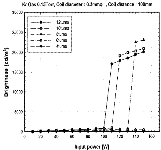
그림 8. 코일의 권선수와 RF 전력 변화에 따른 휘도 특성. Fig. 8. Brightness Dependence on Coil turns and RF power.
