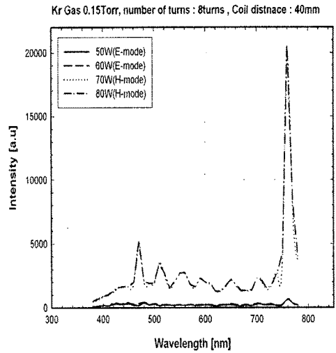
그림 11. RF 전력에 따른 스펙트럼 강도 변화. Fig. 11. Spectrum Intensity Dependence on RF power.
