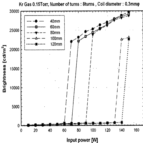
그림 10. 코일의 간격 변화에 따른 휘도 특성. Fig. 10. Brightness Dependence on Coil Distance.
