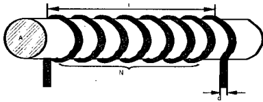
그림 1. 유도결합형 플라즈마 방전관. Fig. 1. Inductively coupled plasma discharge tube.
