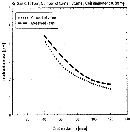
그림 9. 코일의 간격 변화에 따른 인덕턴스 특성. Fig. 9. Inductance Dependence on Coil Distance.
