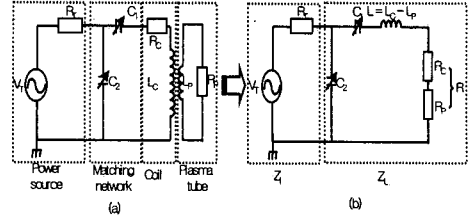
그림 2. 유도결합형 플라즈마 방전관의 전기적인 등가 회로.
