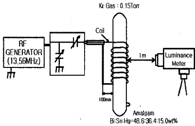
그림 3. 실험 장치 계략도.
