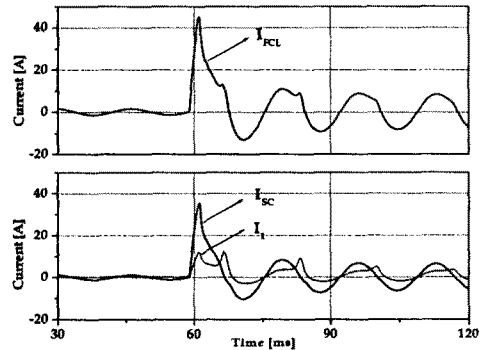
그림 2. 선로전류를 포함한 각 코일의 전류파형
