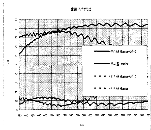
Fig. 1. AZOF 박막의 투과율, 반사율
