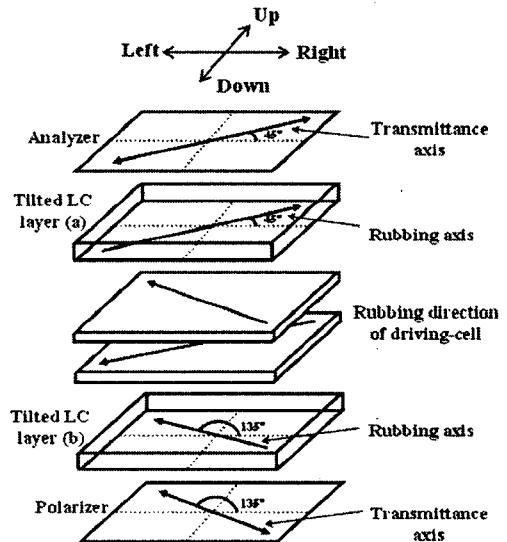
그림 1. 시야각조절 기능을 가진 TN-LCD의 셀 구조.
