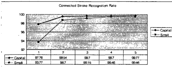
그림 7 영대소문자 5순위 인식률
