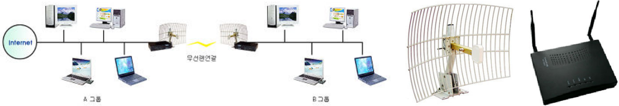
그림 3 브릿지를 이용한 무선랜 구축
