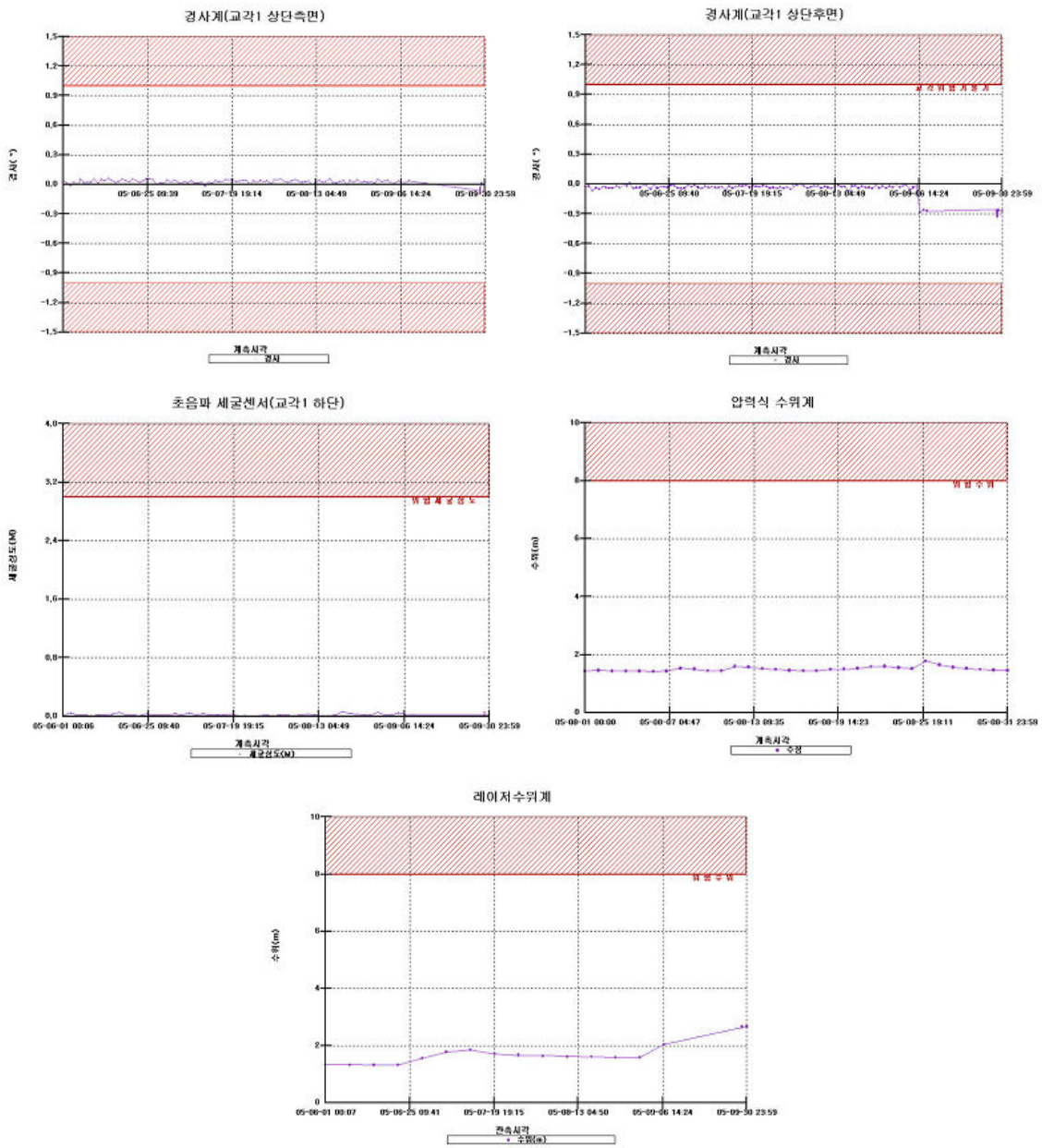
그림 1 센서별 실시간 계측 그래프 예시 (좌상부로부터 교각상단측면 흐름방향 경사계, 교각상단후면 상판방향 경사계, 초음파 세굴센서, 압력식 수위계, 레이저 수위계)
