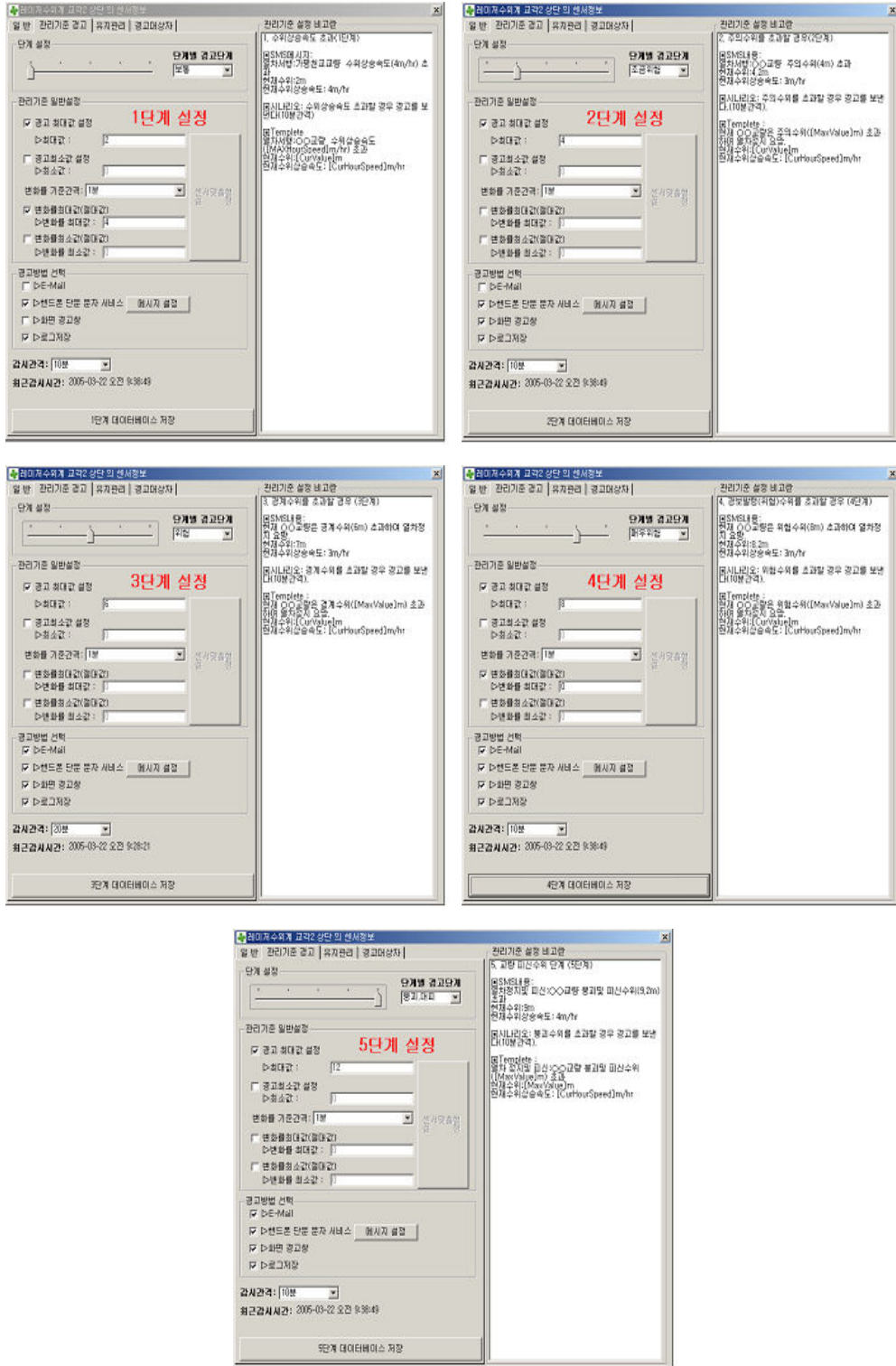
그림 2 조기경보시스템 운영 예 (좌로부터 1단계:수위상승속도 초과, 2단계:주위수위 초과, 3단계:경계수위 초과, 4단계:수위상승속도 초과, 5단계:교량피신수위)
