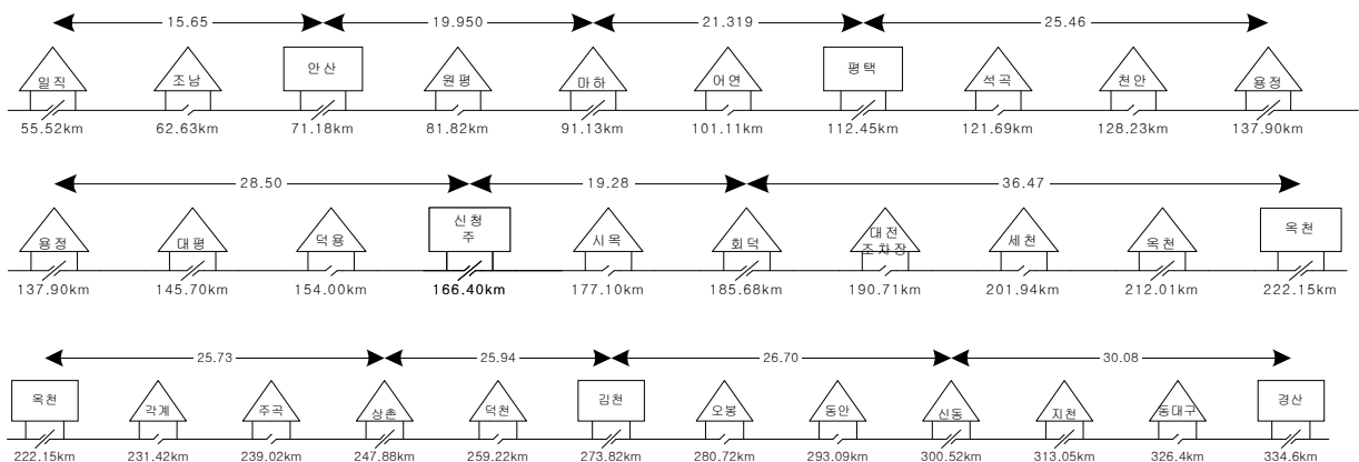
그림 2. 고속철도 운행선로 급전계통도
