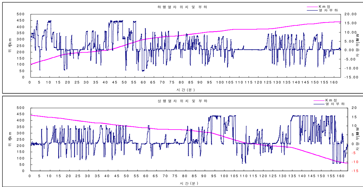
그림 3. 고속열차 열차운행 데이터(추정결과)
