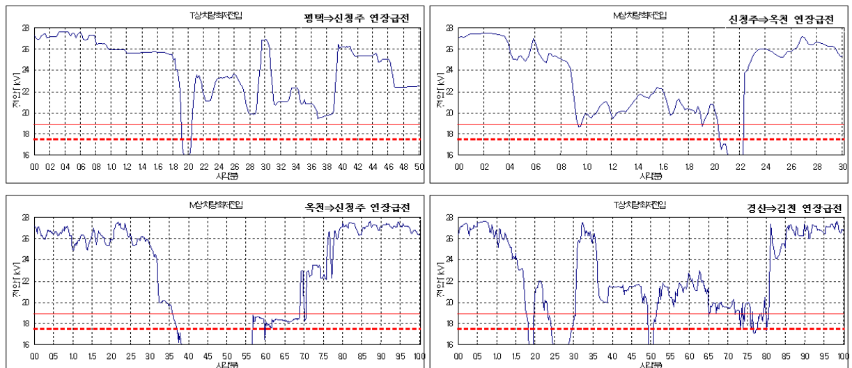
그림 5. 현행 열차운행계획에서 연장급전 최저전압 예측결과
